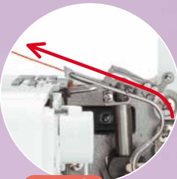
Etape 3 C'est terminé ! La machine a été très simplement enfilée grâce à son enfilage à air. Vous n'aurez plus jamais de difficultés d'enfilage de boucleurs !
